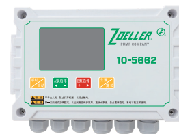
智能控制箱 200 x 140 x 73 mm
