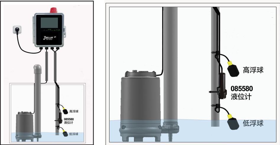
图 5 液位传感器控制
