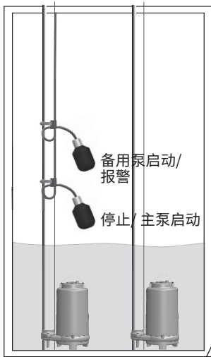
图 1 - 2 浮球控制
