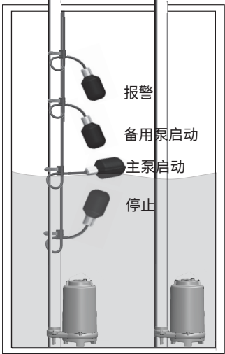
图 3 - 4 浮球控制
