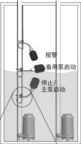
图 2 - 3 浮球控制
