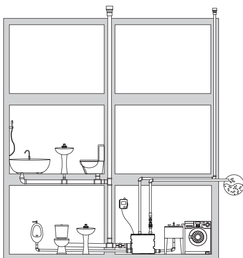
尺寸及安裝示意圖
