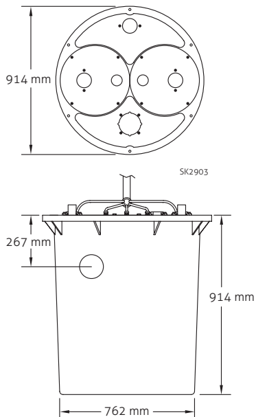
尺寸及安装示意图
