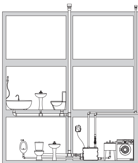
尺寸及安装示意图
