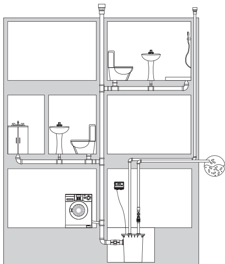
尺寸及安装示意图
